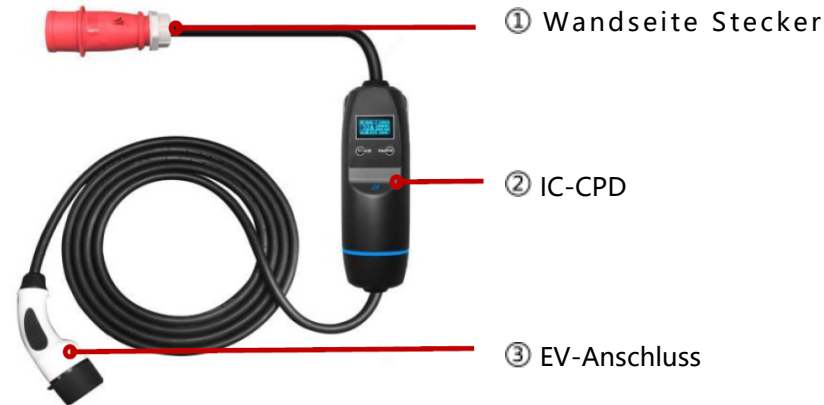
Abbildung 1 Schematische Darstellung
