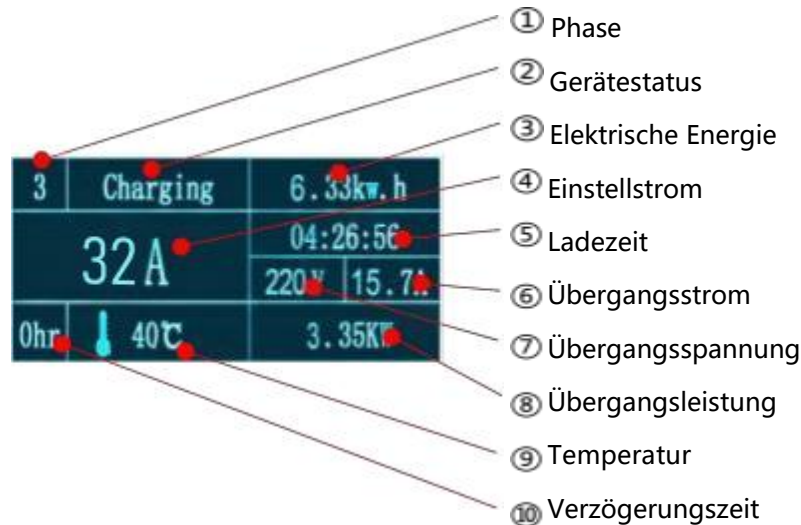
Abbildung 3 Display-Schnittstelle
